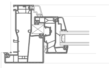
Bovendetail
