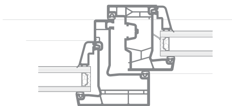
Kalfdetail
